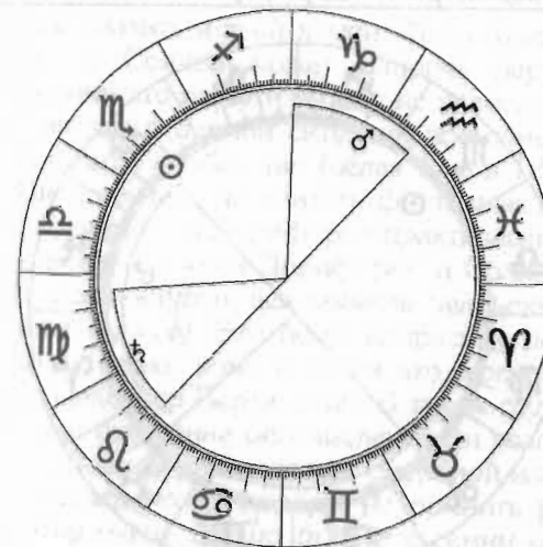
Рис. 12. Расположение Дорифория и Возничего на расстоянии от 48° до 90°.
