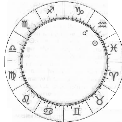
Рис. 7. Марс в роли Дорифория.
