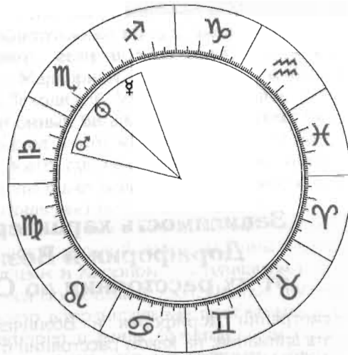
Рис. 10. Расположение Дорифория и Возничего на расстоянии до 28°.
