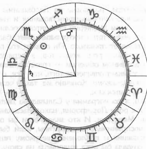
Рис. 11. Расположение Дорифория и Возничего на расстоянии от 28° до 48°.
