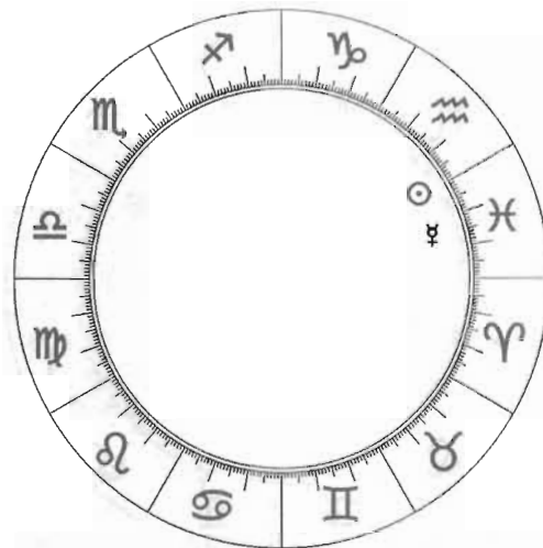
Рис. 8. Меркурий в роли Возничего Солнца.
