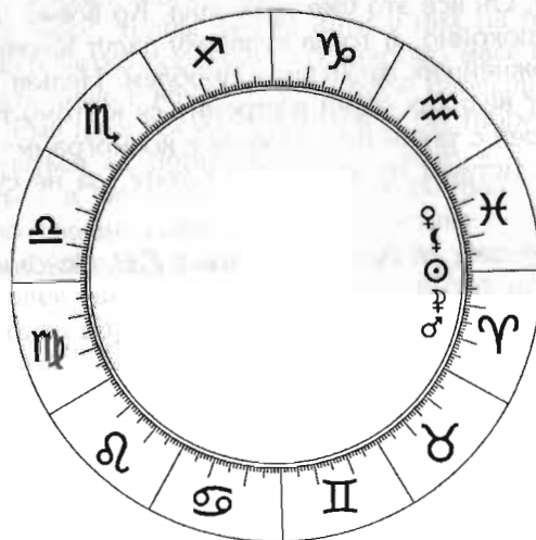
Рис. 9. Фиктивные планеты между Дорифорием и Возничим.
