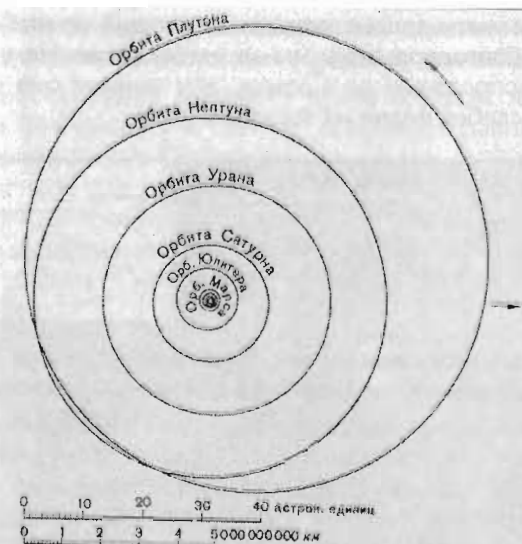
Рис. 2. Строение солнечной системы.
