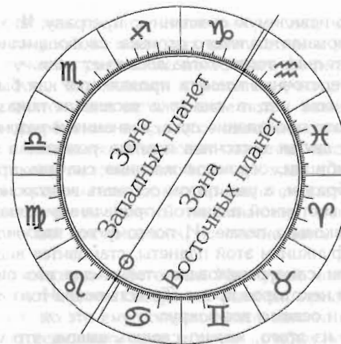
Рис. 5. Разделение Зодиака на две зоны относительно Солнца.
