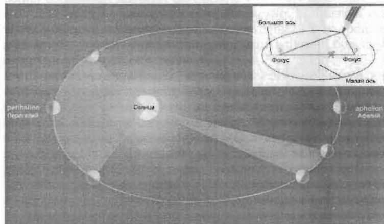
Рис. 3. Схематическое отображение действия законов Кеплера.
