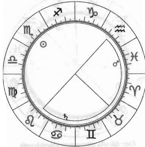
Рис. 13. Расположение Дорифория и Возничего на расстоянии от 90^\circ до 180^\circ .
