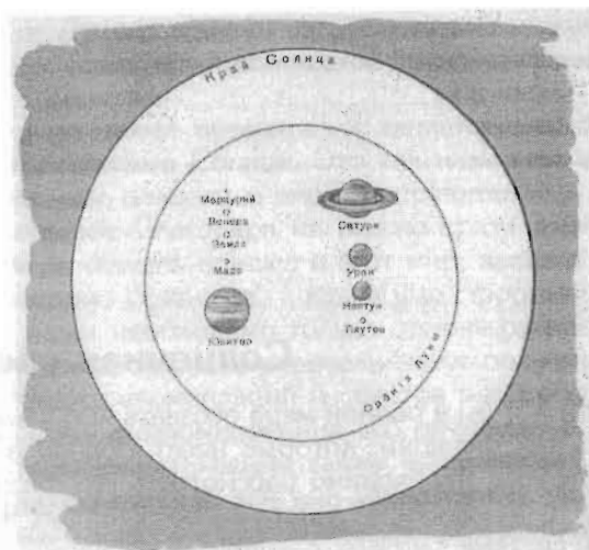
Рис. 1. Сравнительные размеры Солнца и других планет.
