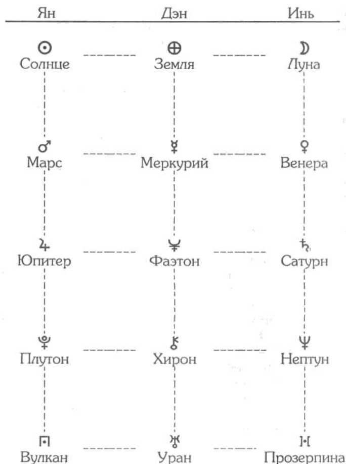
Рис. 3. Планетарная сетка
